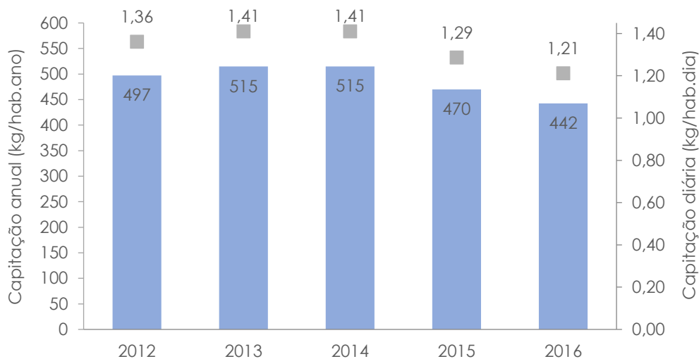
Gráfico 2 - Evolução da produção per capita de resíduos urbanos na ilha de São Jorge
