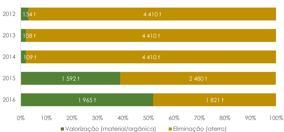
Gráfico 3- Evolução do tratamento de resíduos urbanos na ilha de São Jorge
