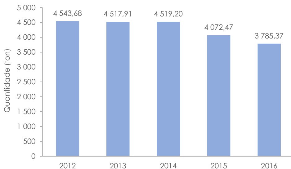
Gráfico 1 - Evolução da produção de resíduos urbanos na ilha de São Jorge
